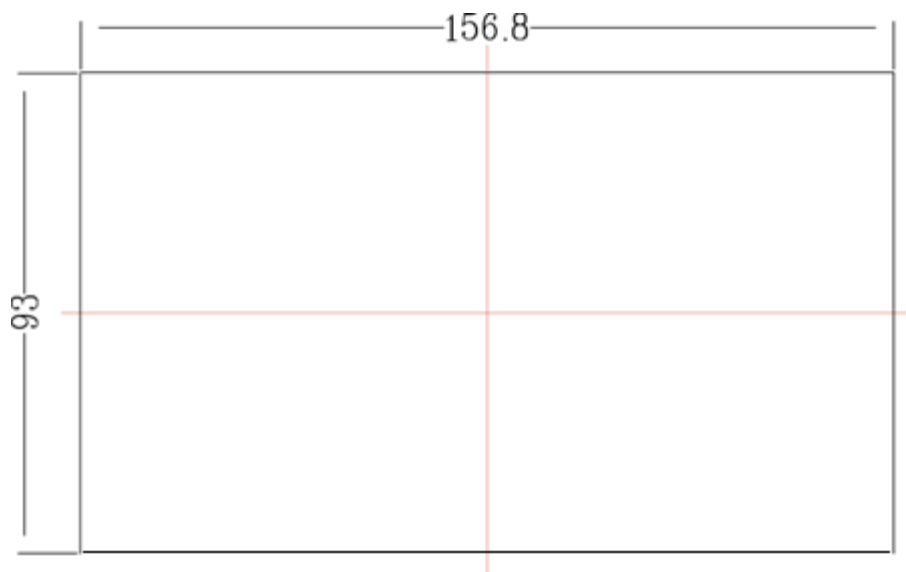
Рис. 25. Размеры отверстия
